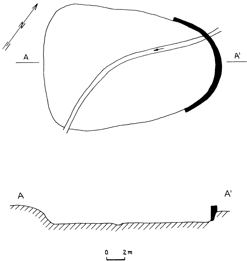
Fig. 86-2. Croquis del estanque de agua en el sitio Cerro La Victoria (AC-86).
